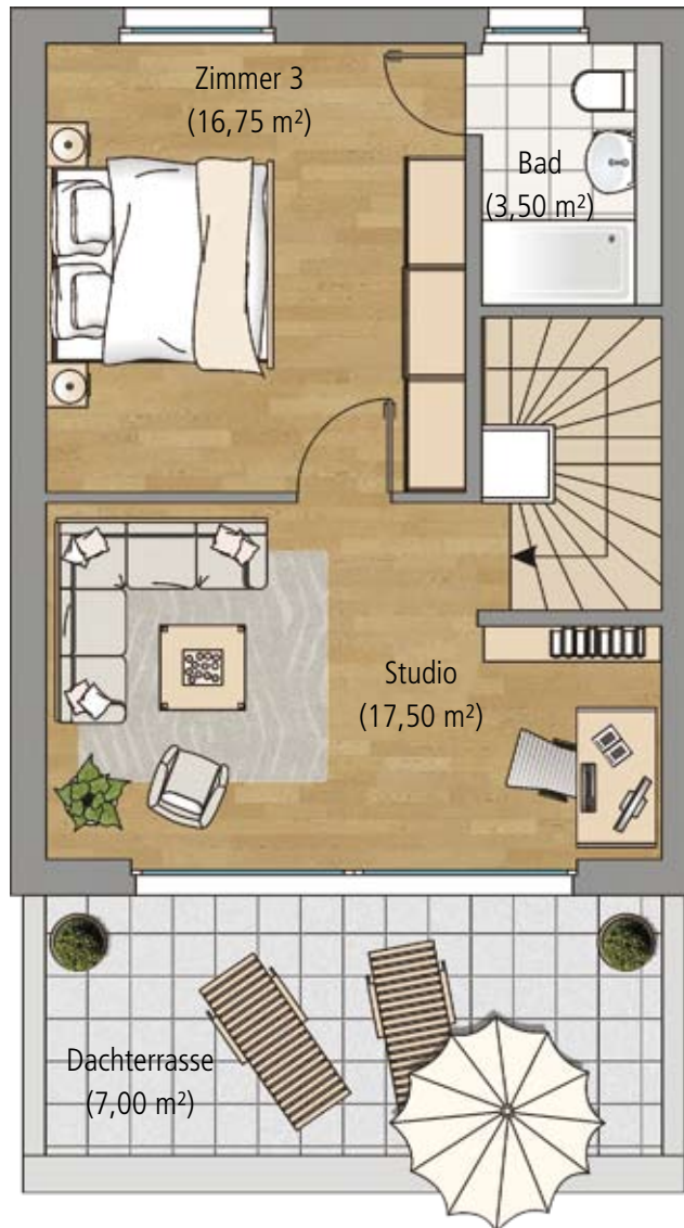
Dachgeschoss Ausbauvariante 1 Haus 2, 4, 8 10, 14 und 16 Haus 3, 5, 9, 11, 15 und 17 sind gespiegelt
